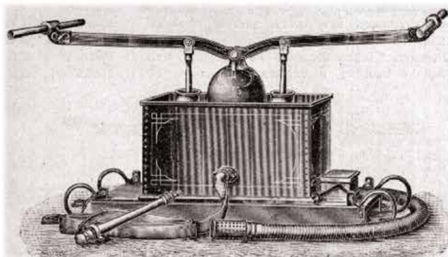
Двухцилиндровая пожарная труба
